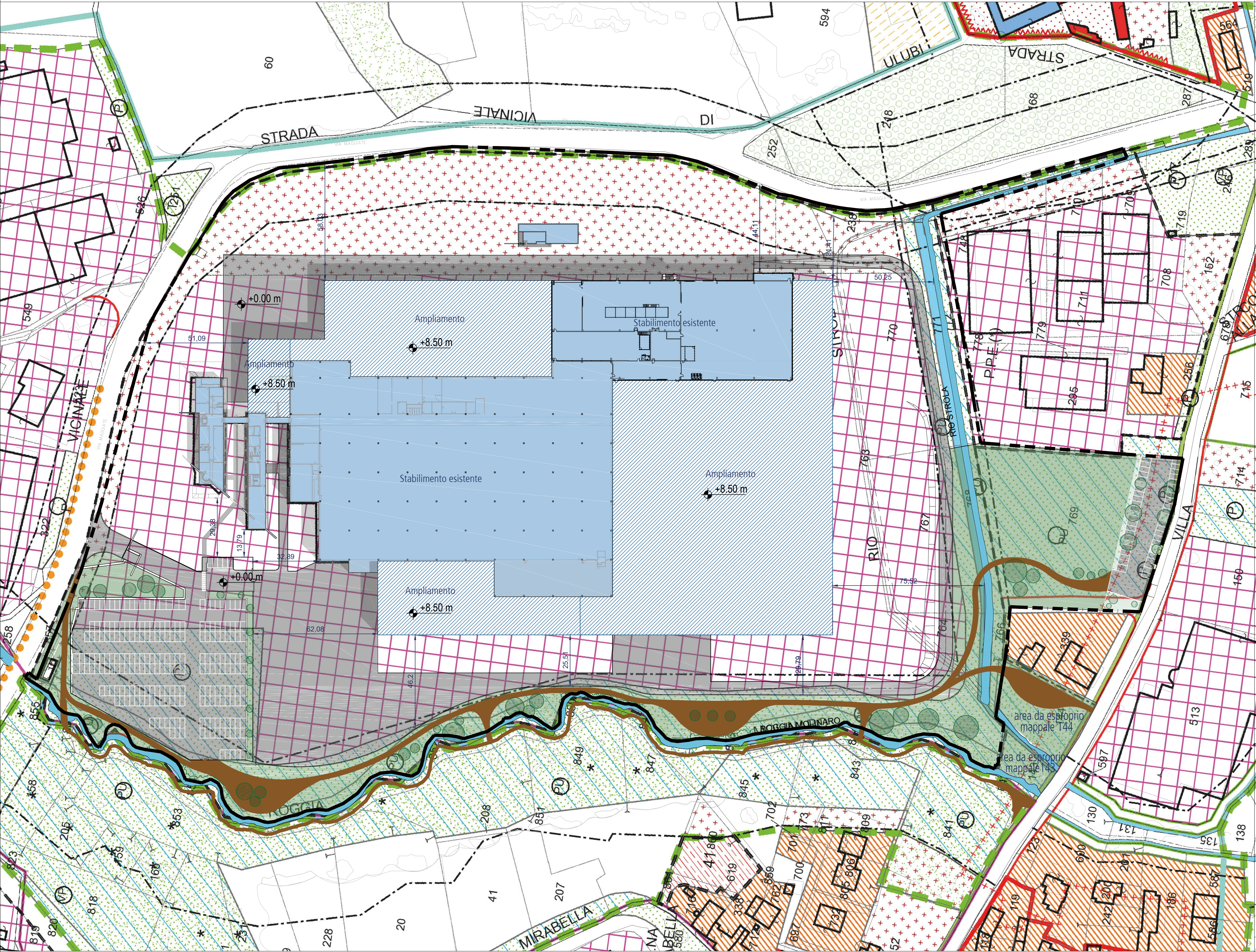
PLANIMETRIA SU BASE DEL P.R.G.C. SC.1:1000
